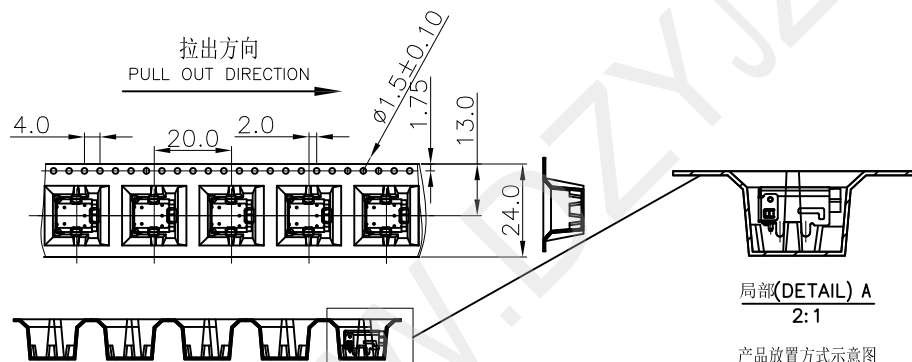
产品放置方式示意图 PLACE PRODUCT AREA
